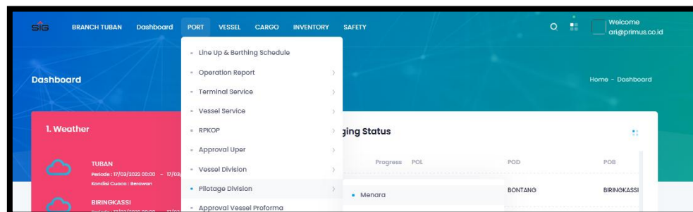
Gambar 50 menu
