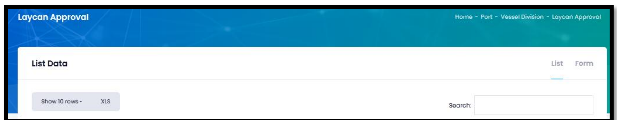
Gambar 9 list laycan
