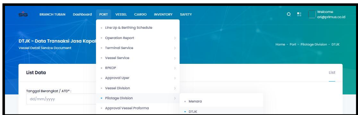
Gambar 59 menu DTJK
